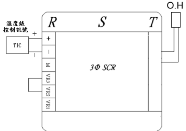
1. 自動模式(4-20mA)
