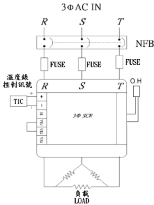
2. 自動(4-20mA)+限制輸出量<->
