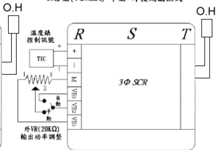
3. 自動(4-20mA)+手動+外接開關模式
